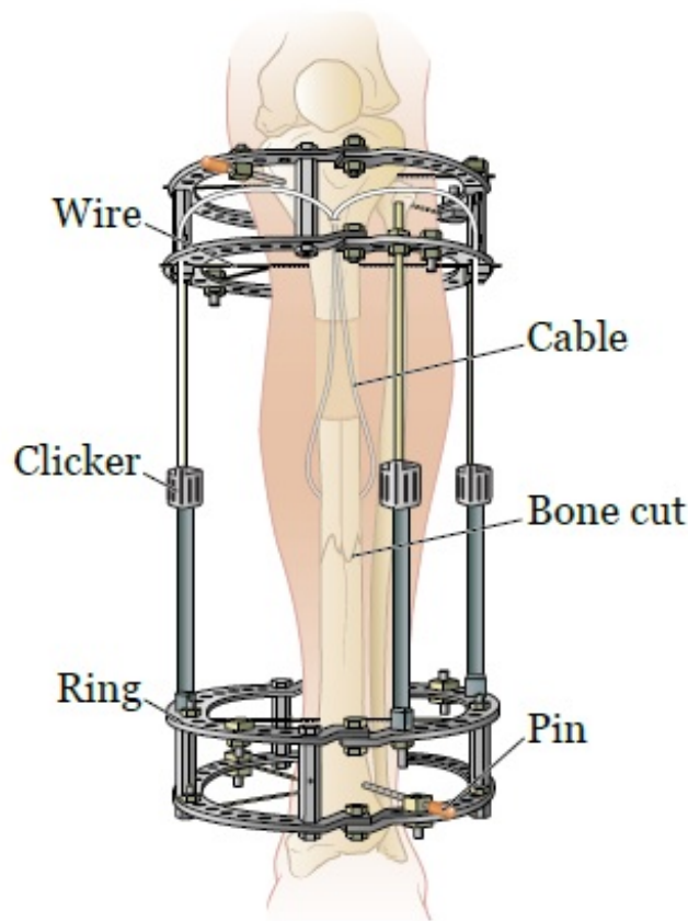
Figura 1. Ejemplo de un fijador externo
