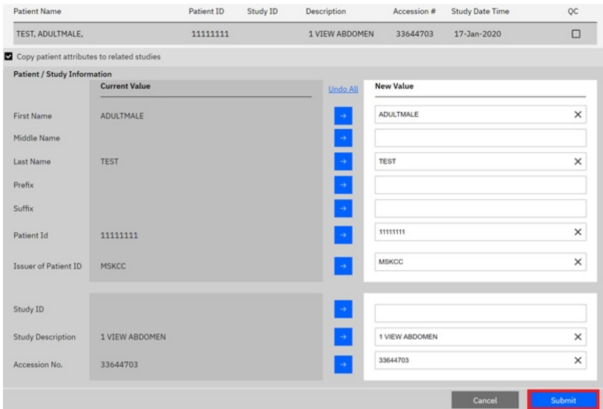
Figura 5. Botón Enviar
