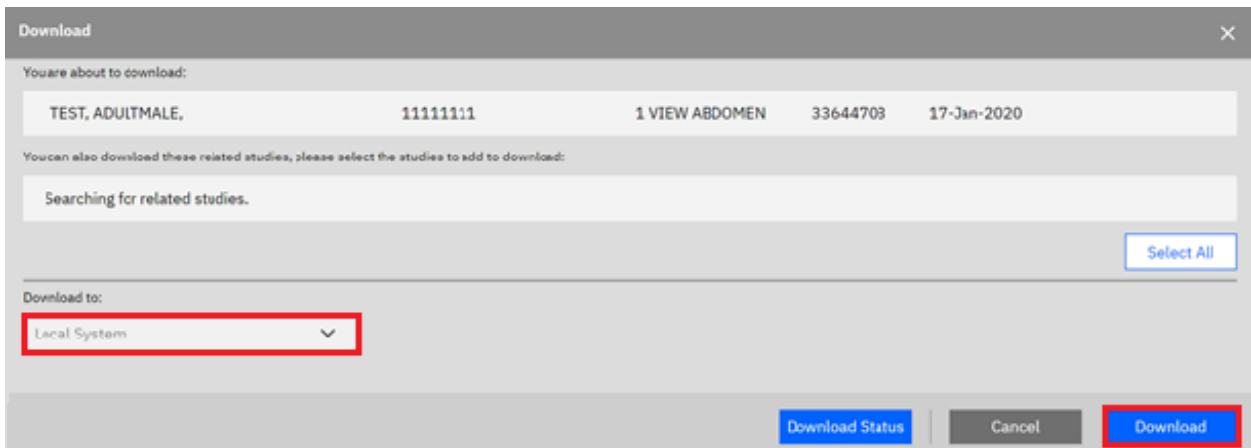
Figura 4. Botón Descargar
