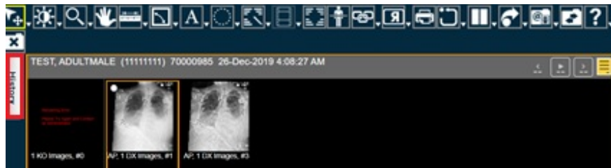
Figura 2. Botón Historial
