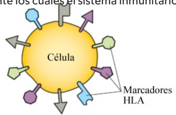
Figura 1. Marcadores HLA
