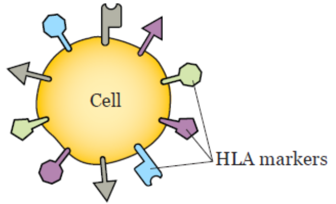
그림 1. HLA 표지자
