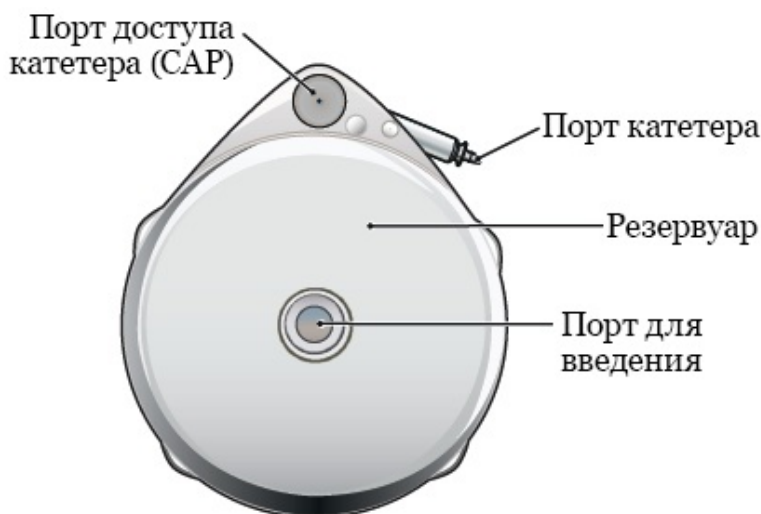
Рисунок 1. Компоненты насоса
