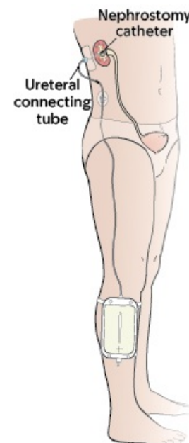
Рисунок 4. Нефростомический катетер
