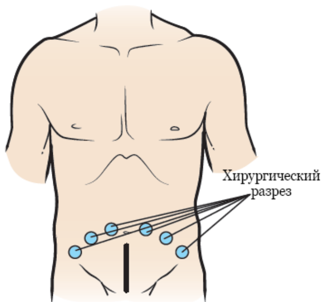
Рисунок 3. Разрезы при лапароскопической или роботизированной простатэктомии
