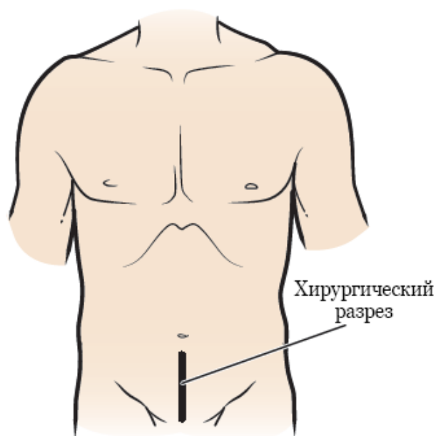
Рисунок 2. Разрез при открытой простатэктомии
