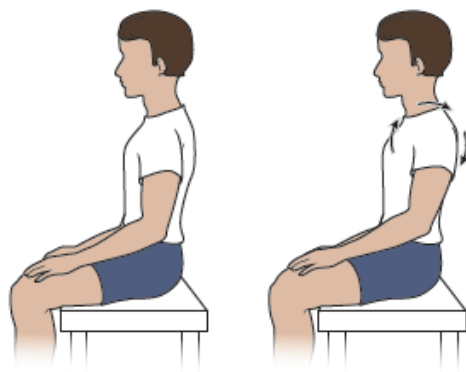
Рисунок 1. Вращение плечами
