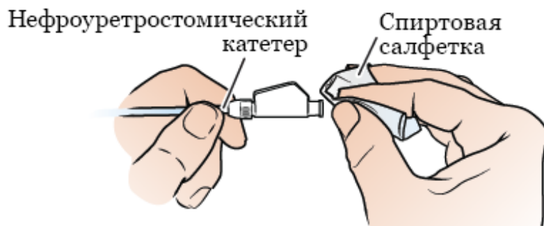
Рисунок 3. Очистка конца катетера
