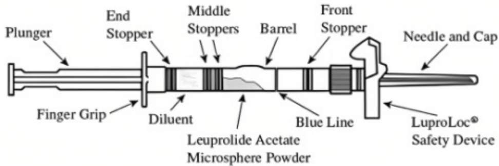
Рисунок 1. Конструкция шприца
