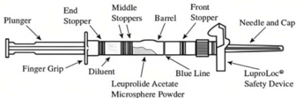
Рисунок 1. Конструкция шприца
