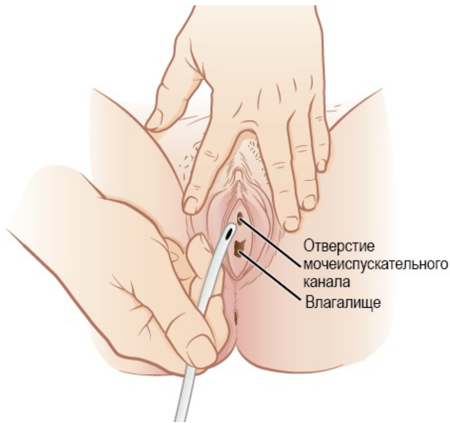
Рисунок 2. Введение катетера
