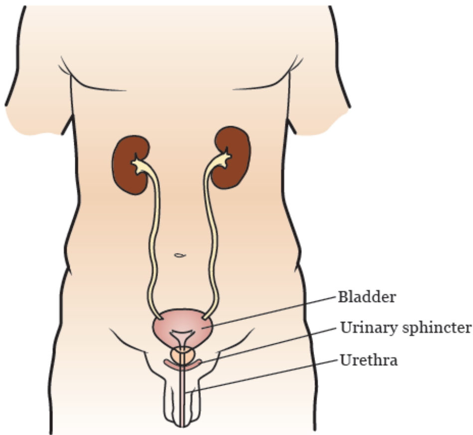
图 1. 尿道括约肌
