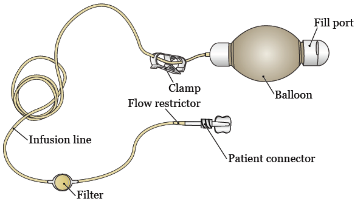
圖 1. 彈性輸液泵的零件
